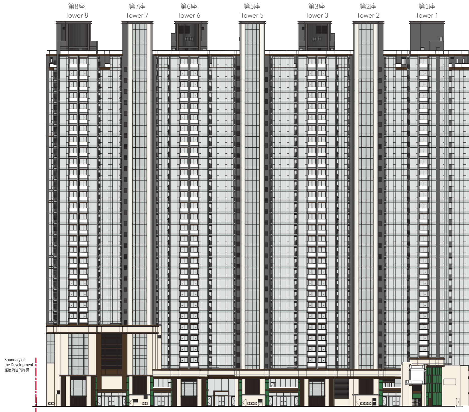
立面圖 2 Elevation 2
